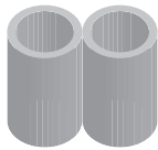
Hole Ø14mm/ External Ø18mm/ H.30mm
